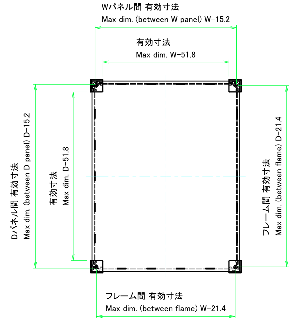
下カバー / Bottom cover
